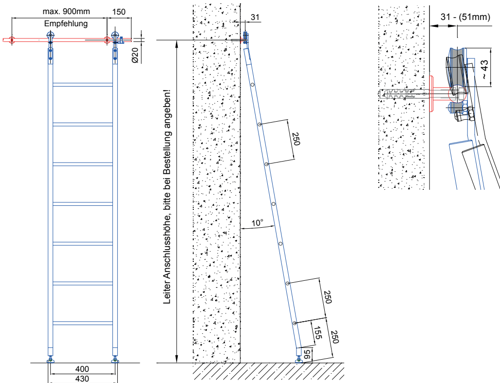
Beispiel Modell SL 6020 Sprossen
