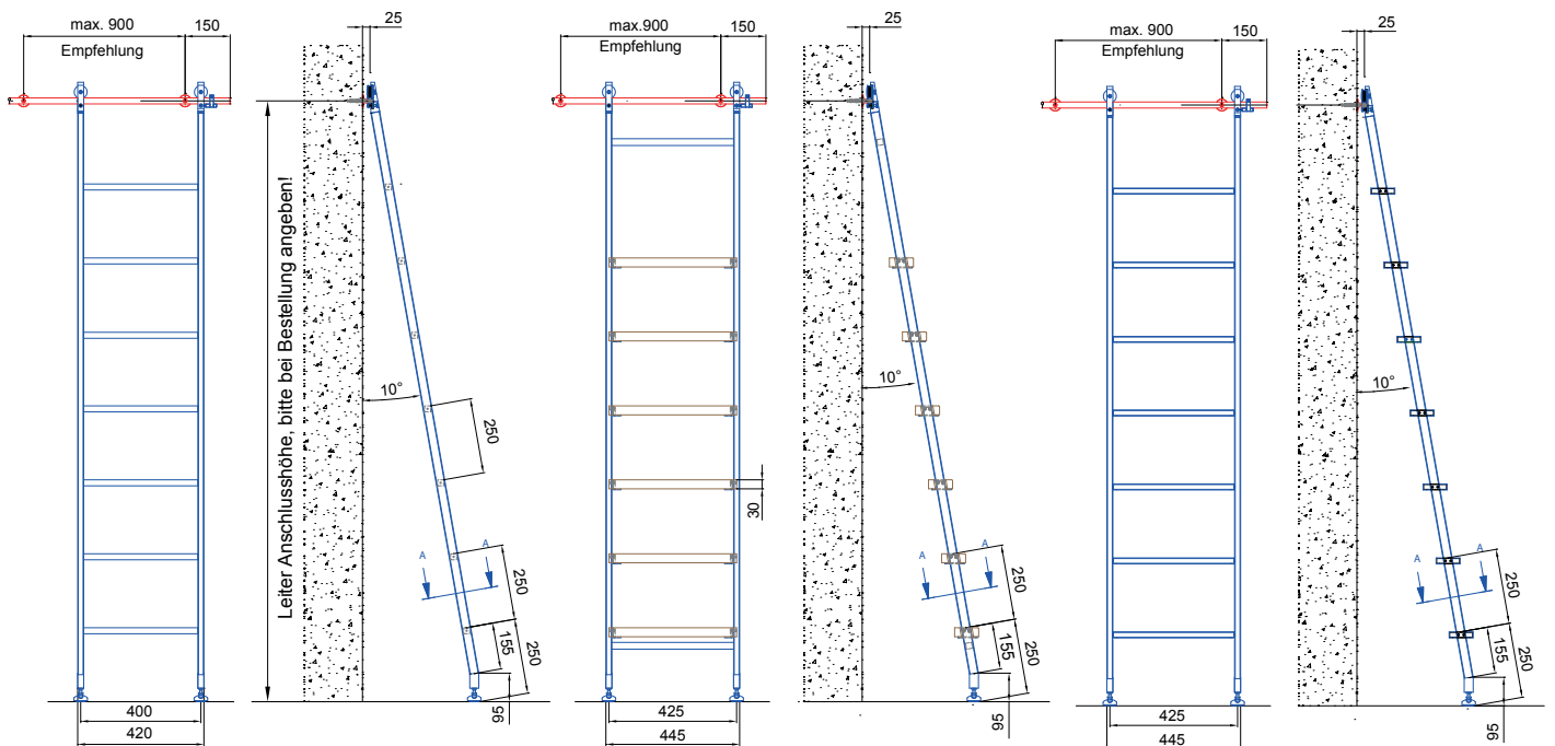
Beispiel Modell SL 6070 mit Edelstahlsprossen
